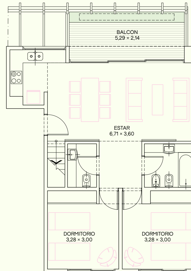
PLANTA BAJA
